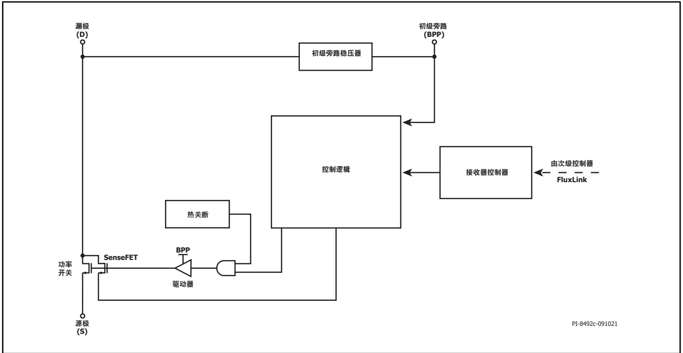
图 3. 初级控制器框图
